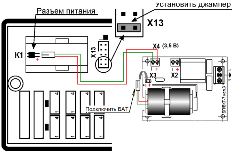
Рис. И.3 Схема подключения БП к ВКГ-3Т
