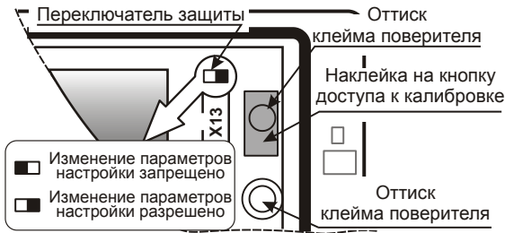
Рис. 3.1а – Места пломбирования поверителем
