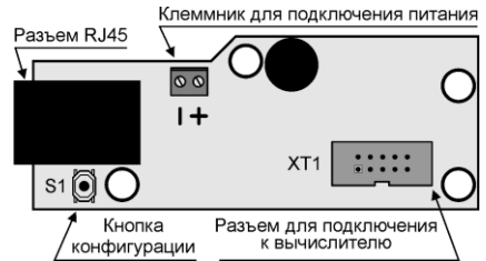
Рис. К.1 – Внешний вид платы адаптера Ethernet
