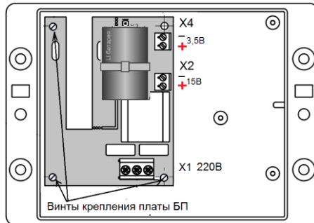
Рис. И.2 – Схема монтажа БП в корпусе
