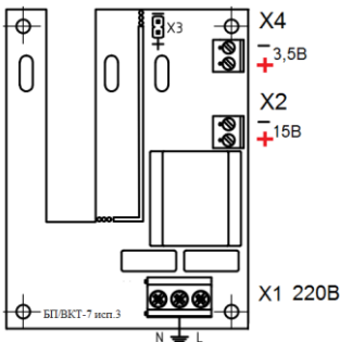
Рис. И.1 Внешний вид БП/ВКТ-7
