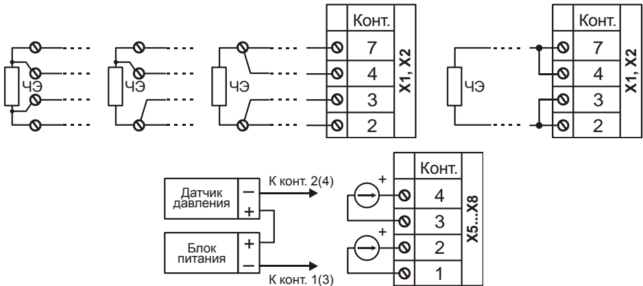
Рис. 5.2 – Подключение ТС и ДД к вычислителю
