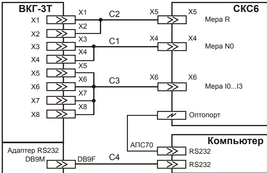
Рисунок 7.1 – Схема поверки
