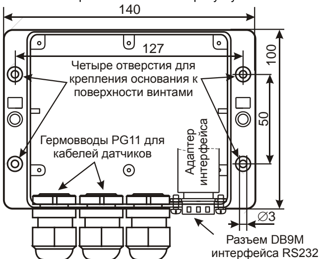
Рисунок 5.1 – Схема крепления вычислителя
